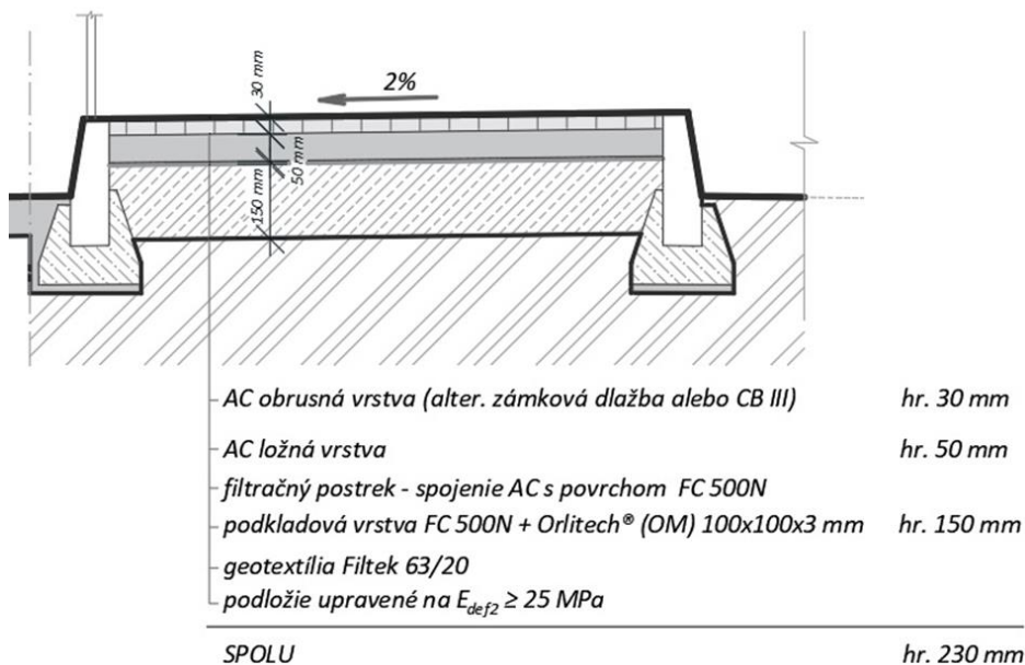
Obr. 2 Príklad návrhu skladby chodníka s povolenými 7 prejazdmi TNV / 24 hod
