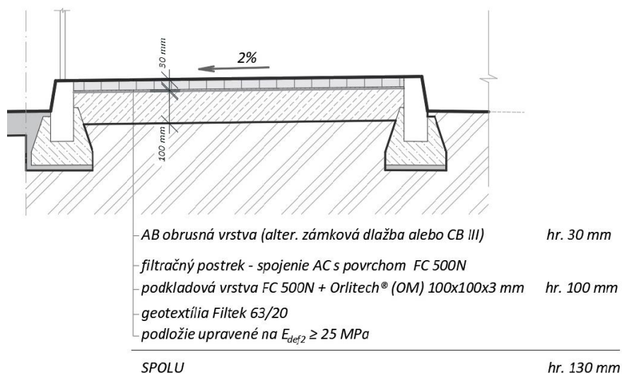
Obr. 1 Príklad nízkonákladového návrhu skladby chodníka s úplne vylúčenou nákladnou dopravou
